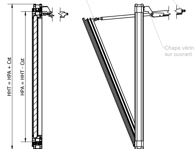
B-B ( 1:10 )
